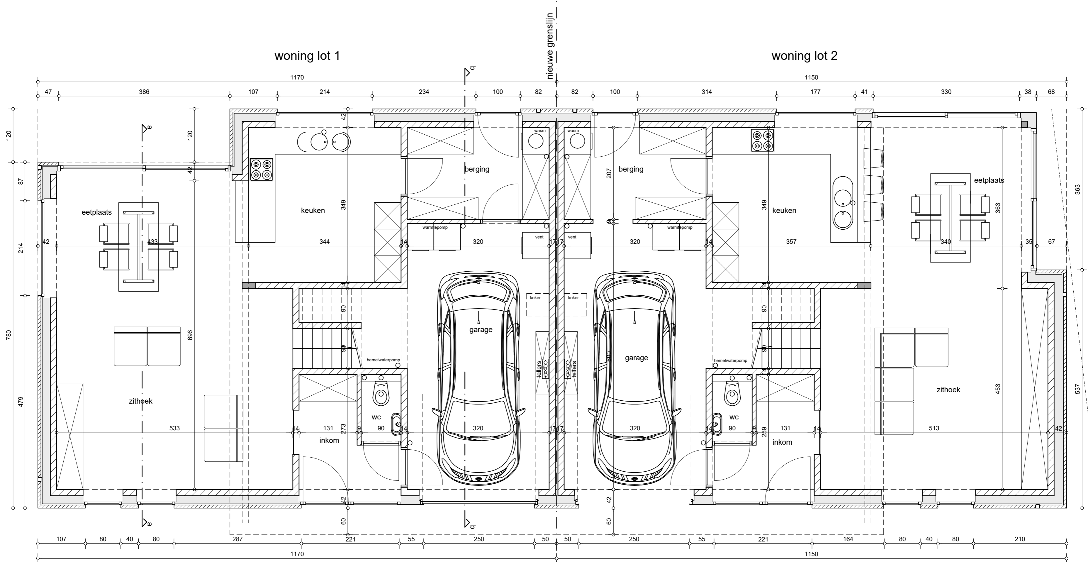
grondplan
